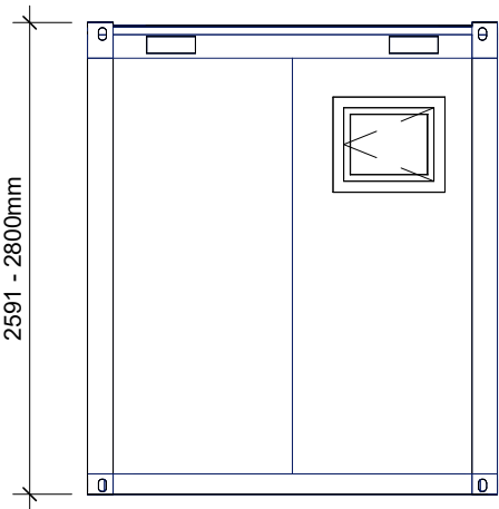
Ansicht Ost
