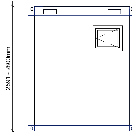
Ansicht Ost
