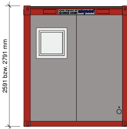
Ansicht Ost
