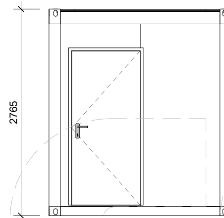
Ansicht West
