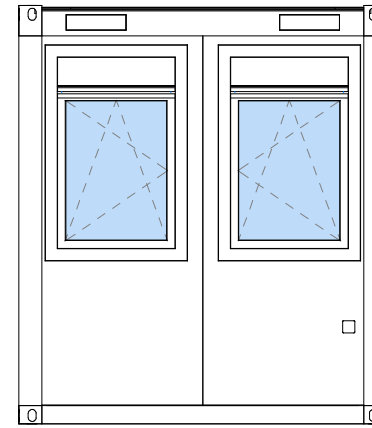
Ansicht Ost
