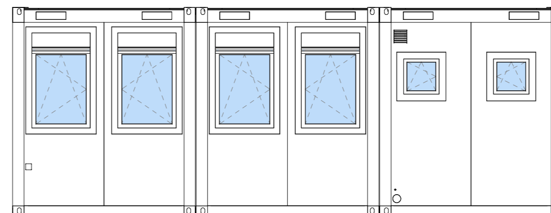
Ansicht Ost
