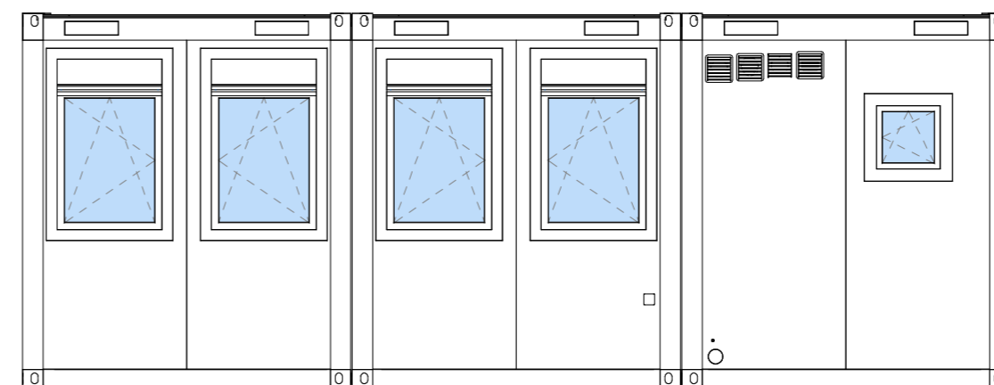
Ansicht Ost
