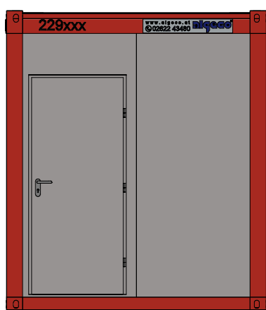
Ansicht West
