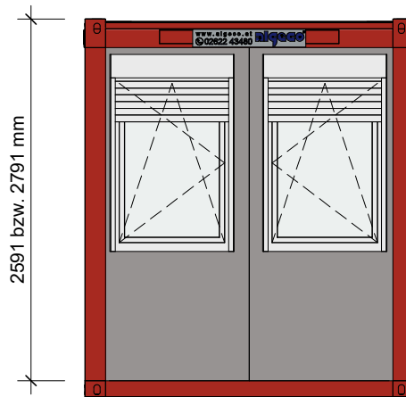
Ansicht Ost
