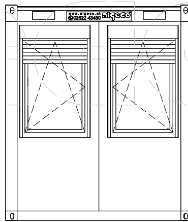
Ansicht Ost
