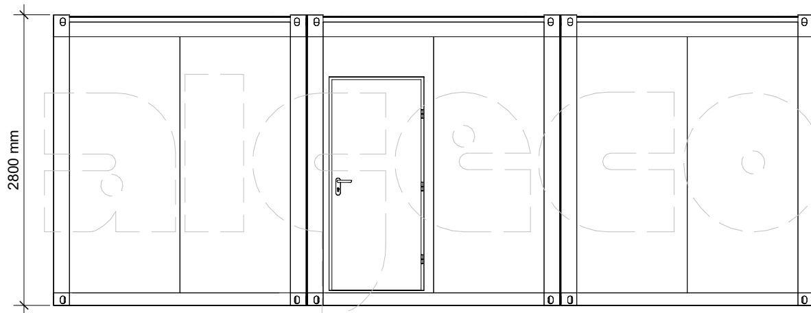
Ansicht West
