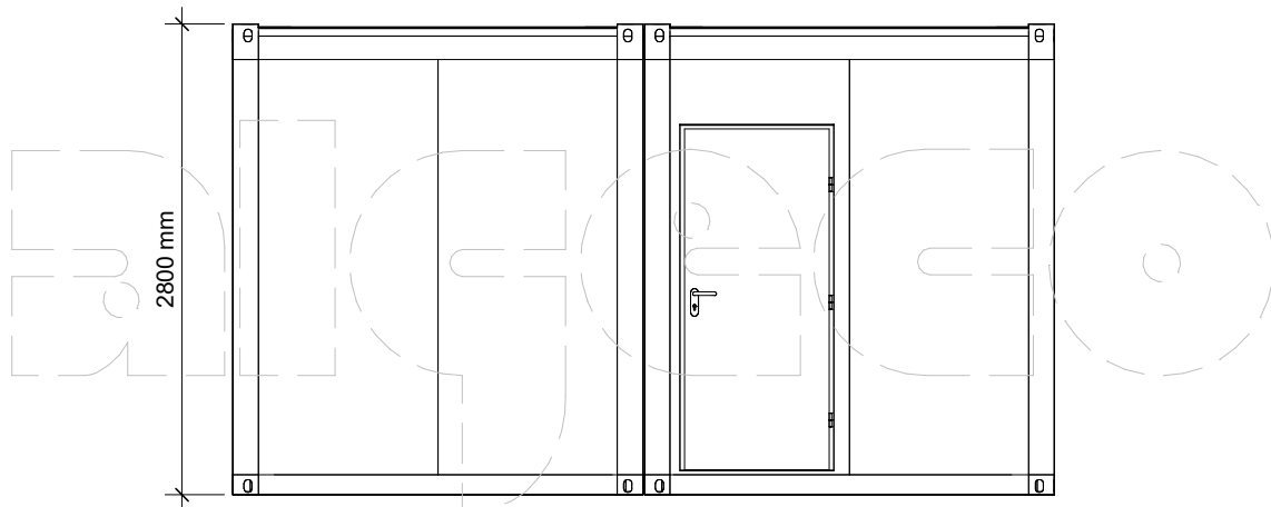
Ansicht West
