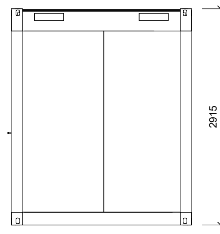
Ansicht Ost
